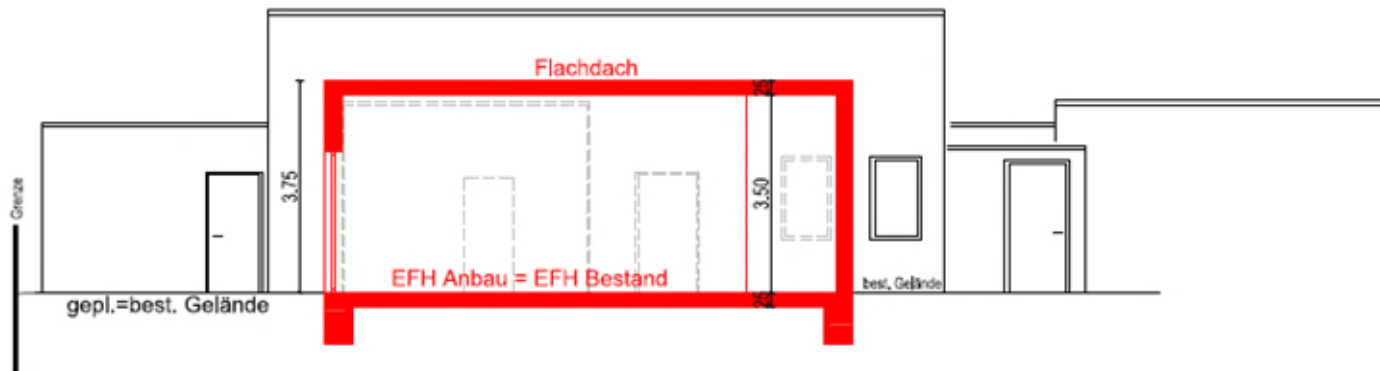
Schnitt A-A
